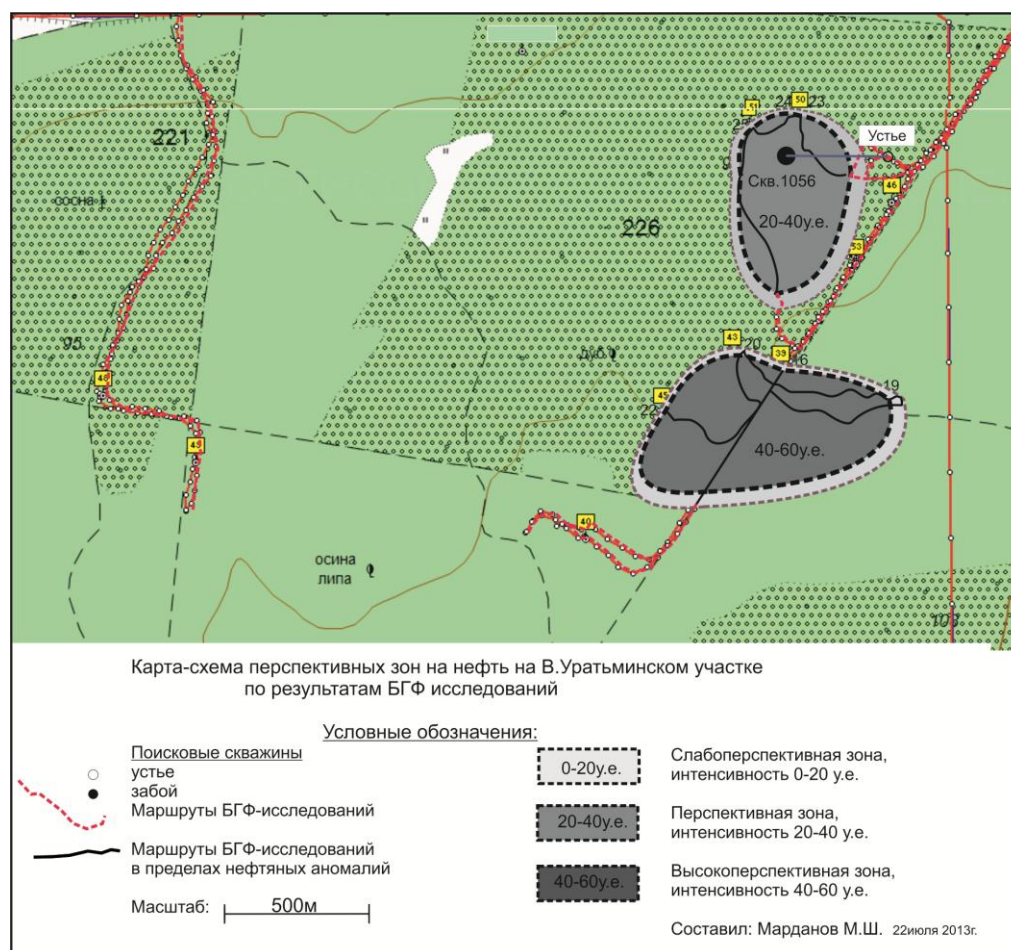
Рис.4 Карта-схема по результатам БГФ-исследований на Уртымском участке.
