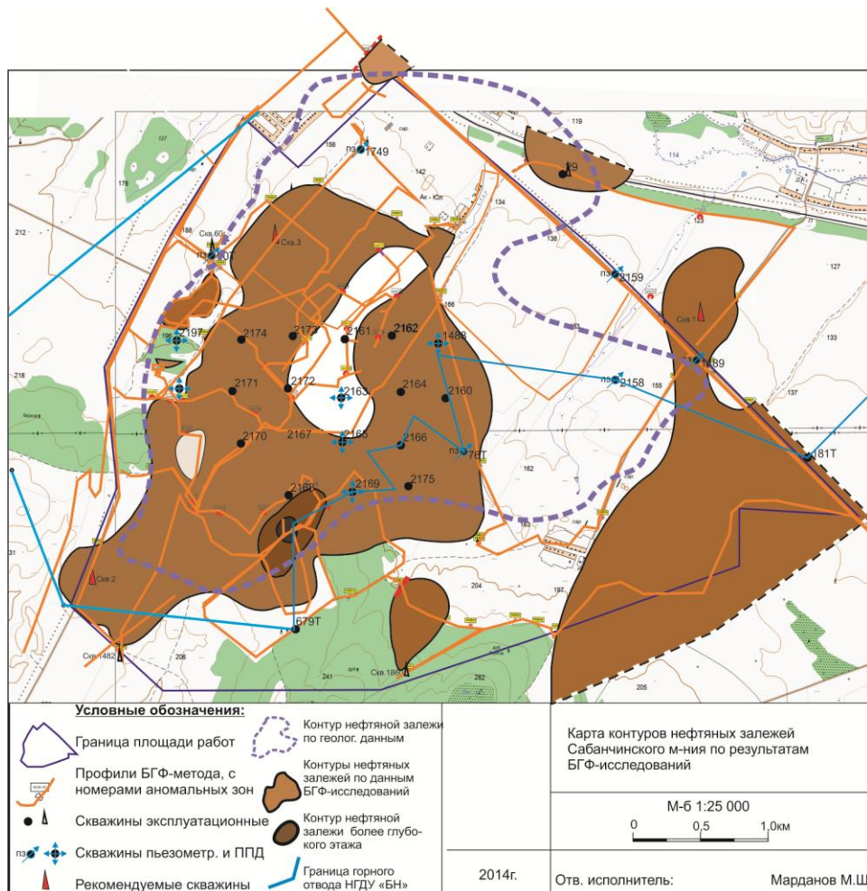
Рис.6 Результаты работ БГФ-методом на Сабанчинском нефтяном месторождении.
