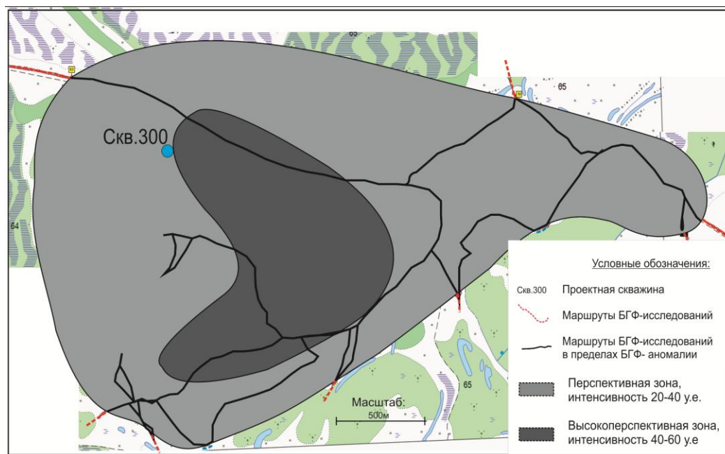
Рис.5 Результаты исследований БГФ-методом на Тлянчи-Тамакском участке.
