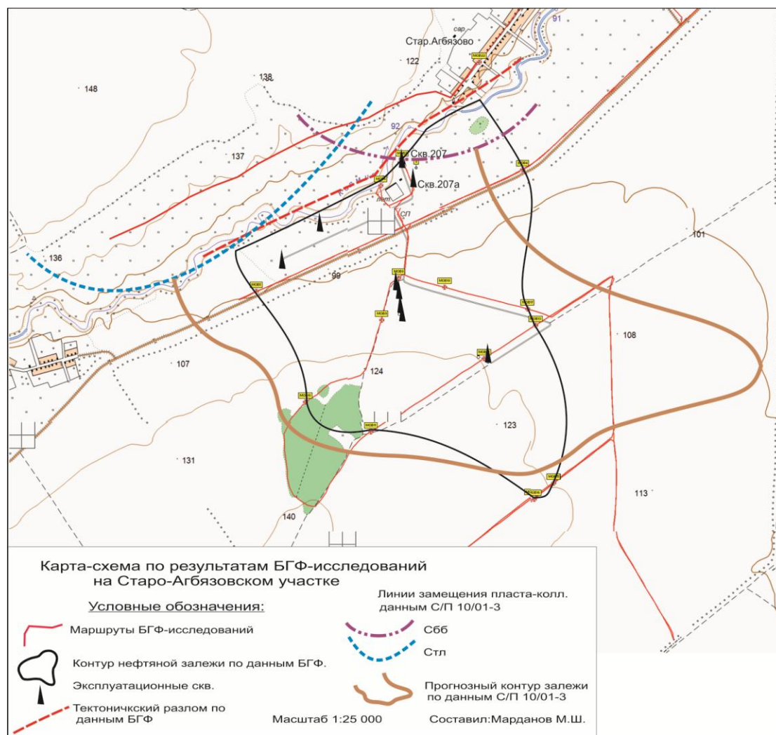
Рис. 3 Результаты БГФ-исследований на Старо-Агбязовском участке.
